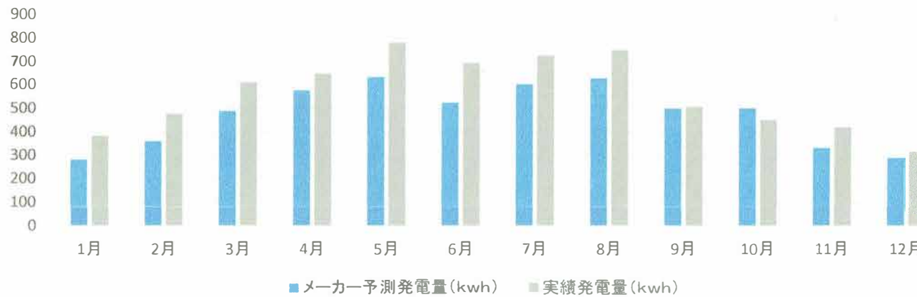
発電量比較
